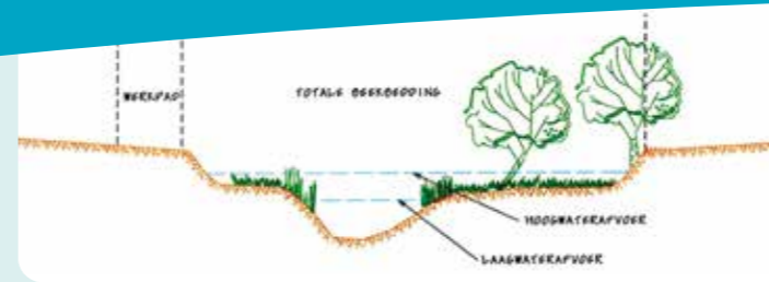
Natuurlijk herstel van de beekbedding verlaagt het overstromingsrisico.
